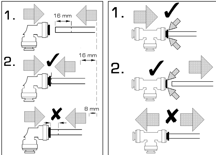
Fig 6 – RACCORDS – Branchement et Débranchement
